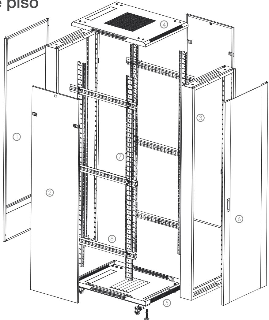
CARACTERÍSTICAS TÉCNICAS GABINETES PISO ESTÁNDAR
